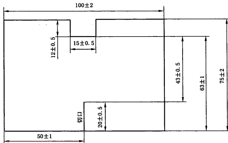
图 1 试样尺寸图
